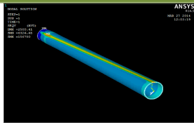
VON MISES ANALYSIS FOR HM-CARBON EPOXY
